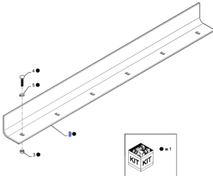
Listwa bębna podajnika łapacz kamieni 1324437C1
