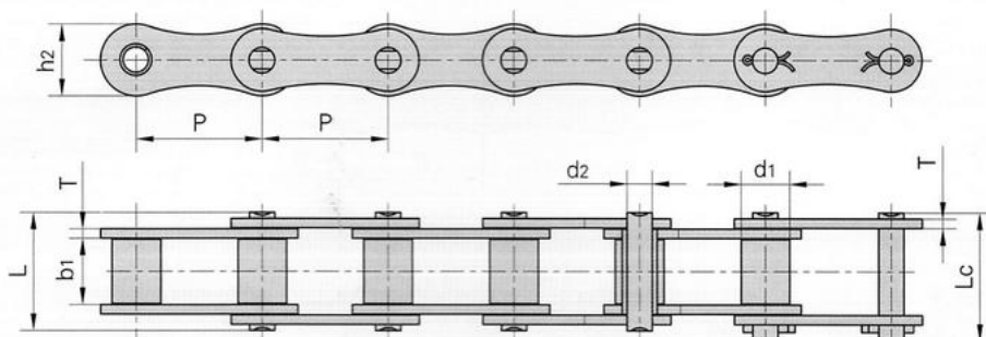
Łańcuch rolkowy Claas 32S
